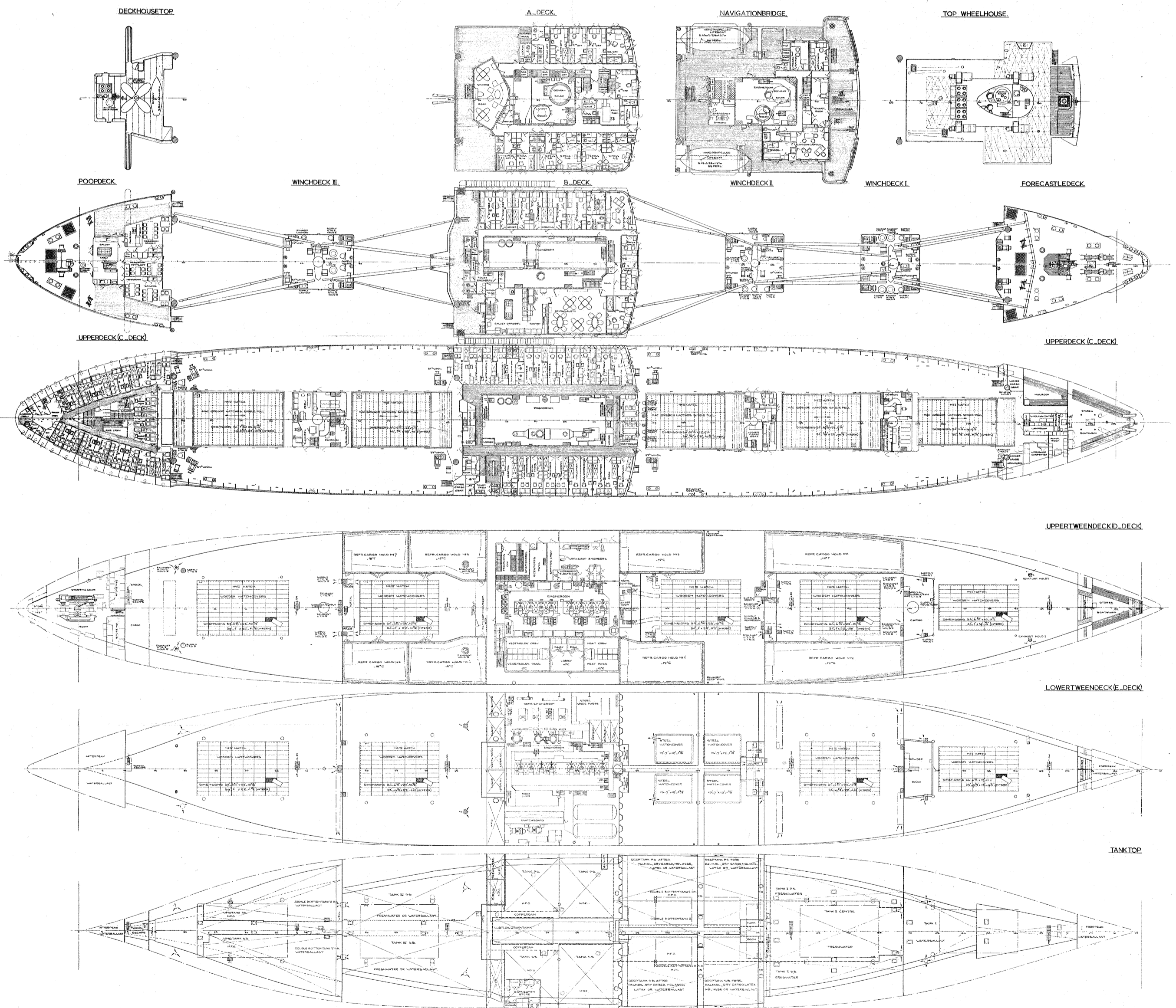
M.S. „STRAAT MAGELHAEN” Algemeen plan en dekkenplan
